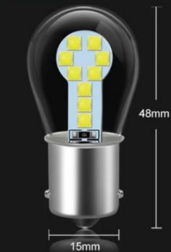
BA15S
